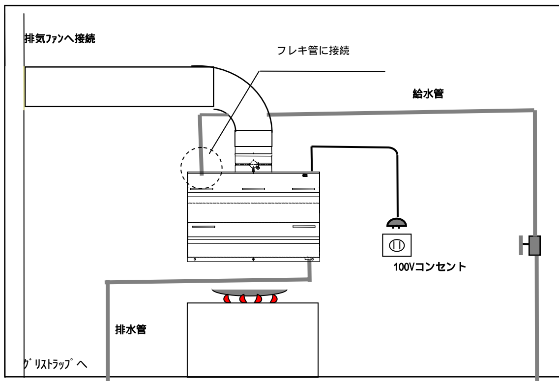
図7 . 配管工事例
