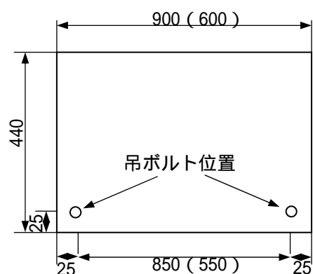
吊ボルト位置
