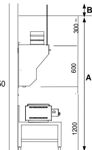
吊ボルト寸法
