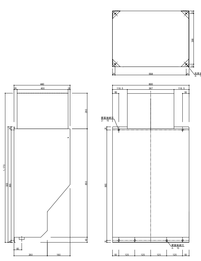
図6 . KC62-FR 取付寸法図
