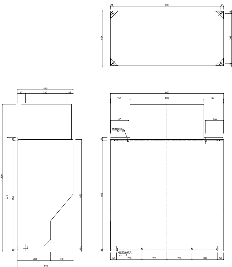
図5 . KC92-FR 取付寸法図
