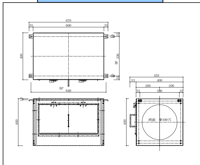
PCF5-20型外形寸法図
