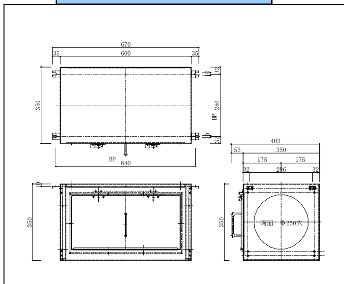
PCF5-10型外形寸法図
